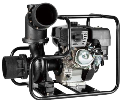
Модель БНЦ-6д-100м³/ч-15м-ЭС
