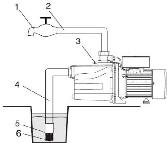
Правильная установка.
