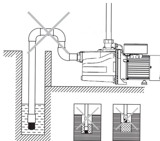
Неправильная установка.
