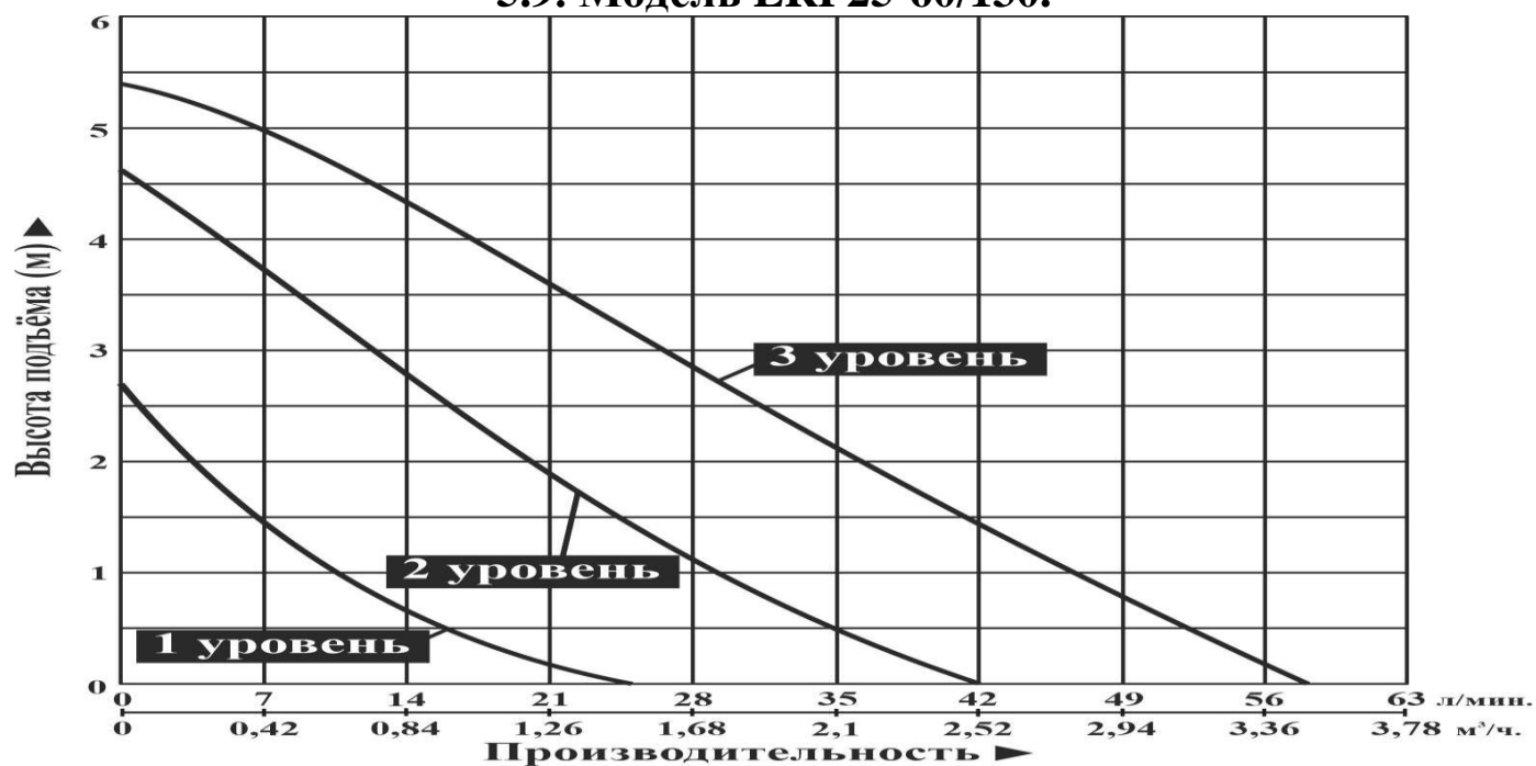
5.9. Модель LRP25-60/130.
